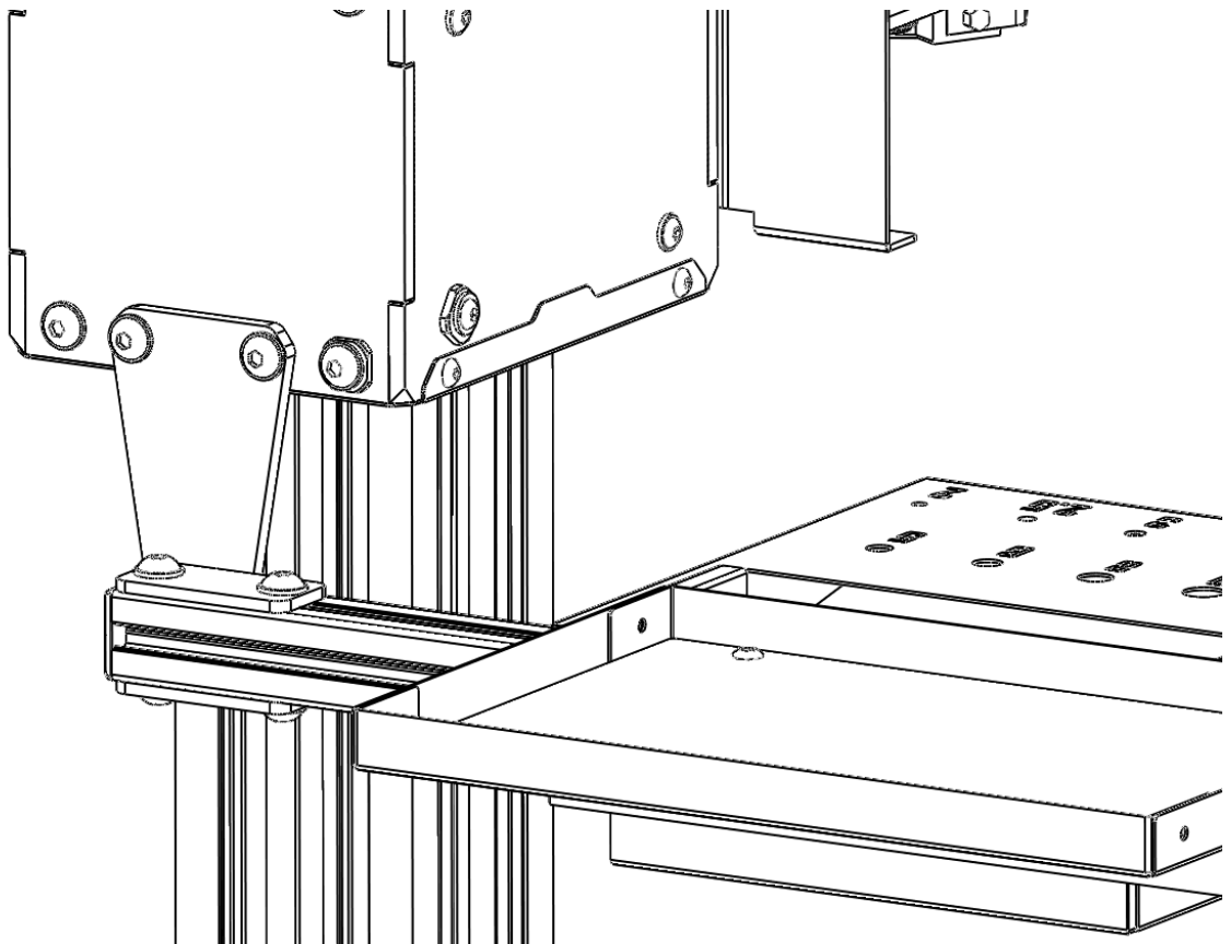
Figuur 2: Bevestiging van de vaste arm
