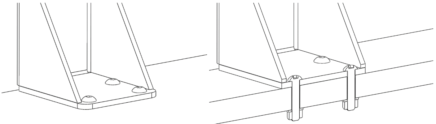
Montage met schroefdraad / profielweergave
