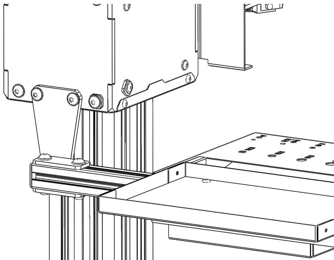
Figura 2: Montaggio a braccio fisso
