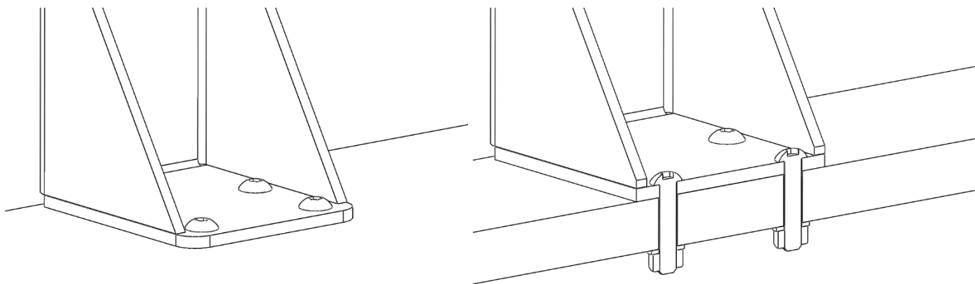
Montaggio con viti filettate / vista a sezione
