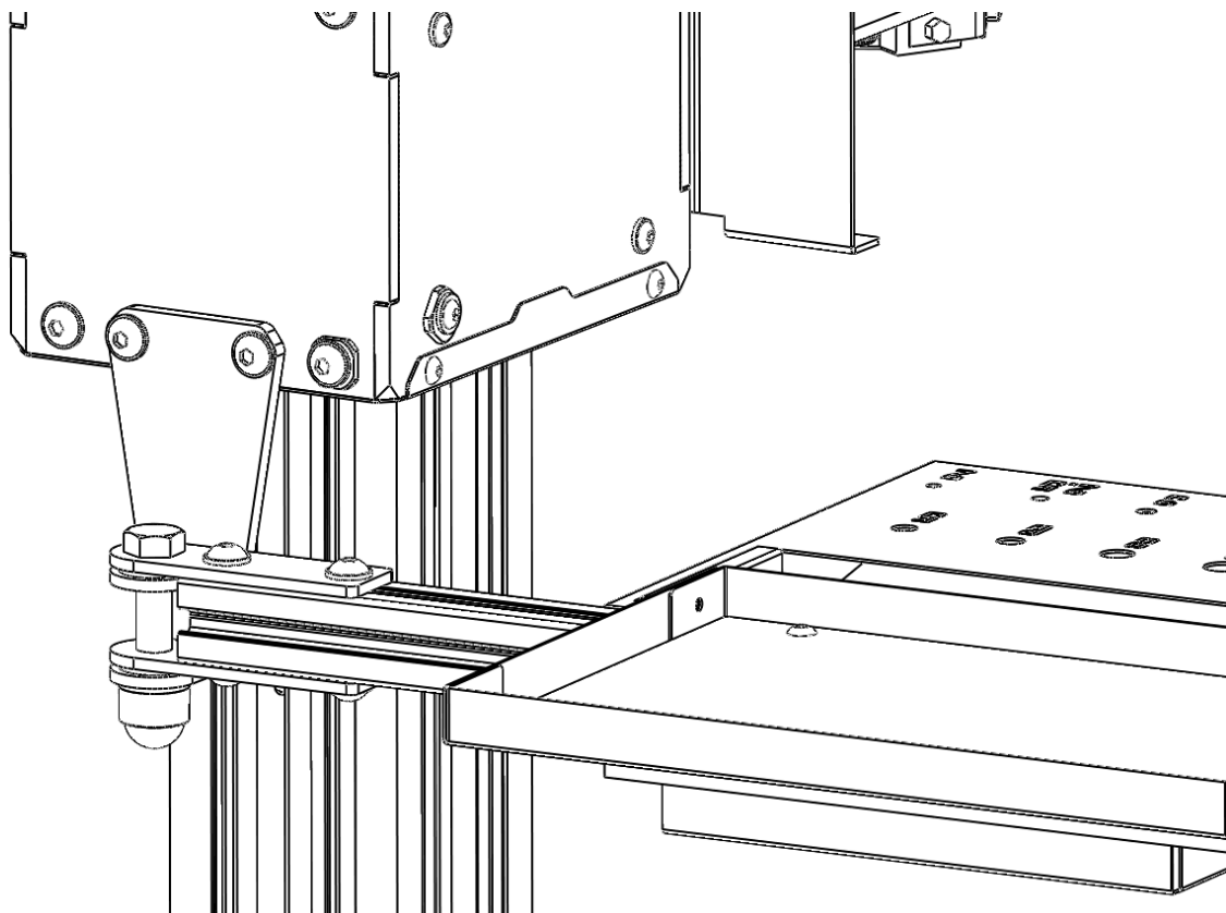
Figura 1: Montagem do braço articulado
