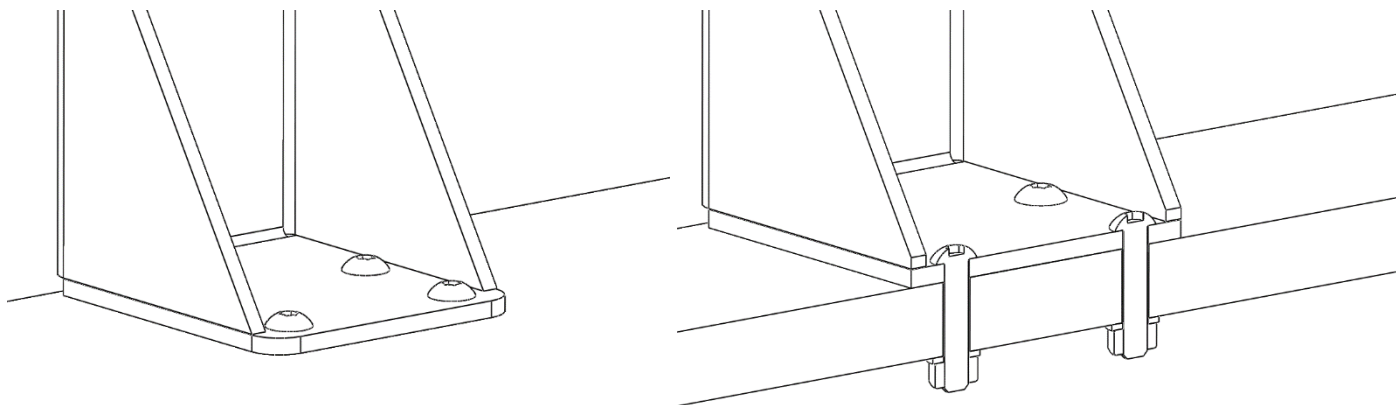
Montagem com parafusos roscados / vista de secção
