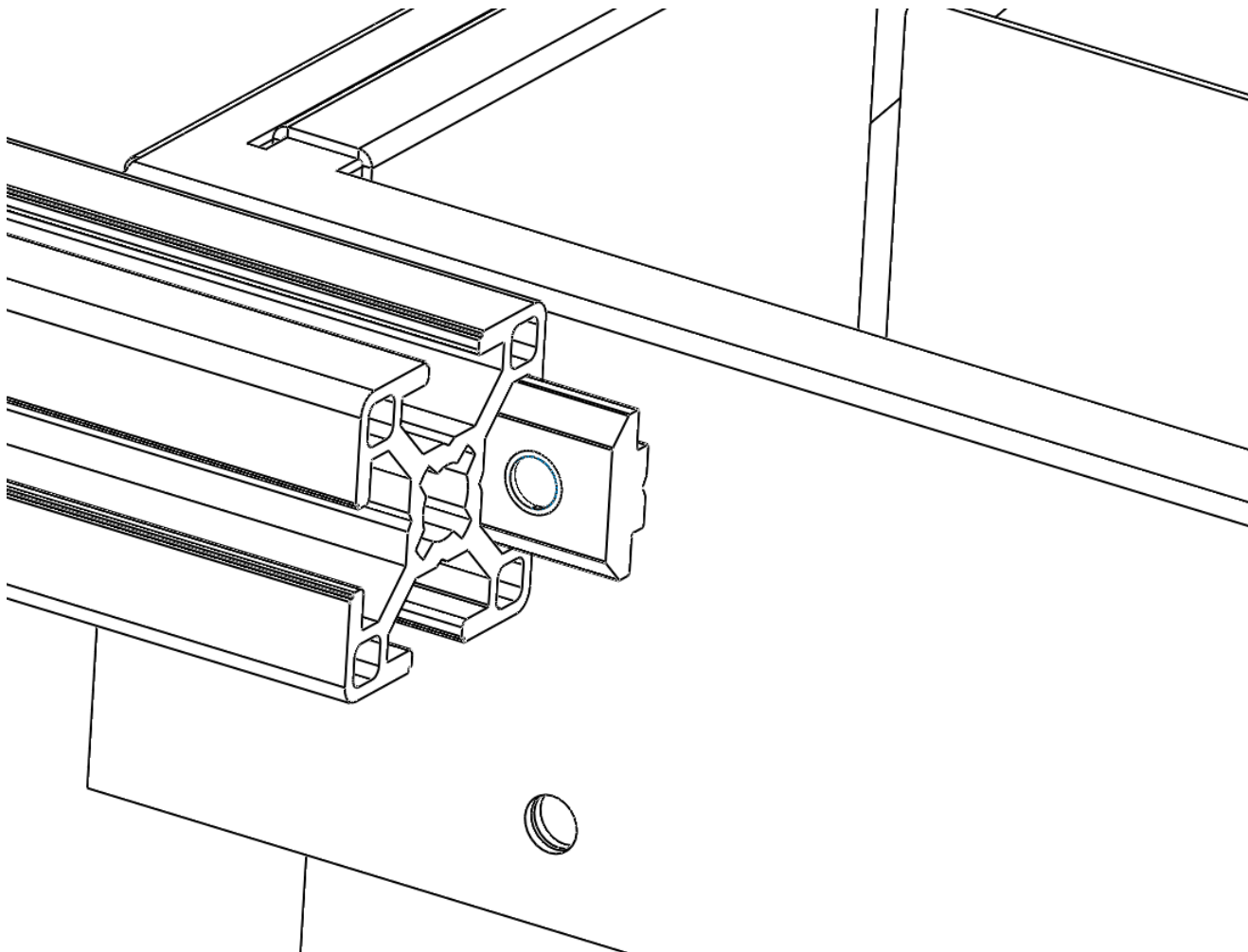
Figur 8: Monteringsdetalje for værktøjsbakke
