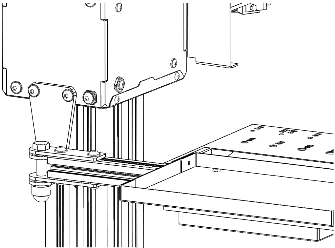
Figur 1: Hængslet armmontering
