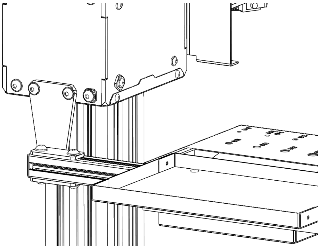
Figur 1: Hængslet armmontering
