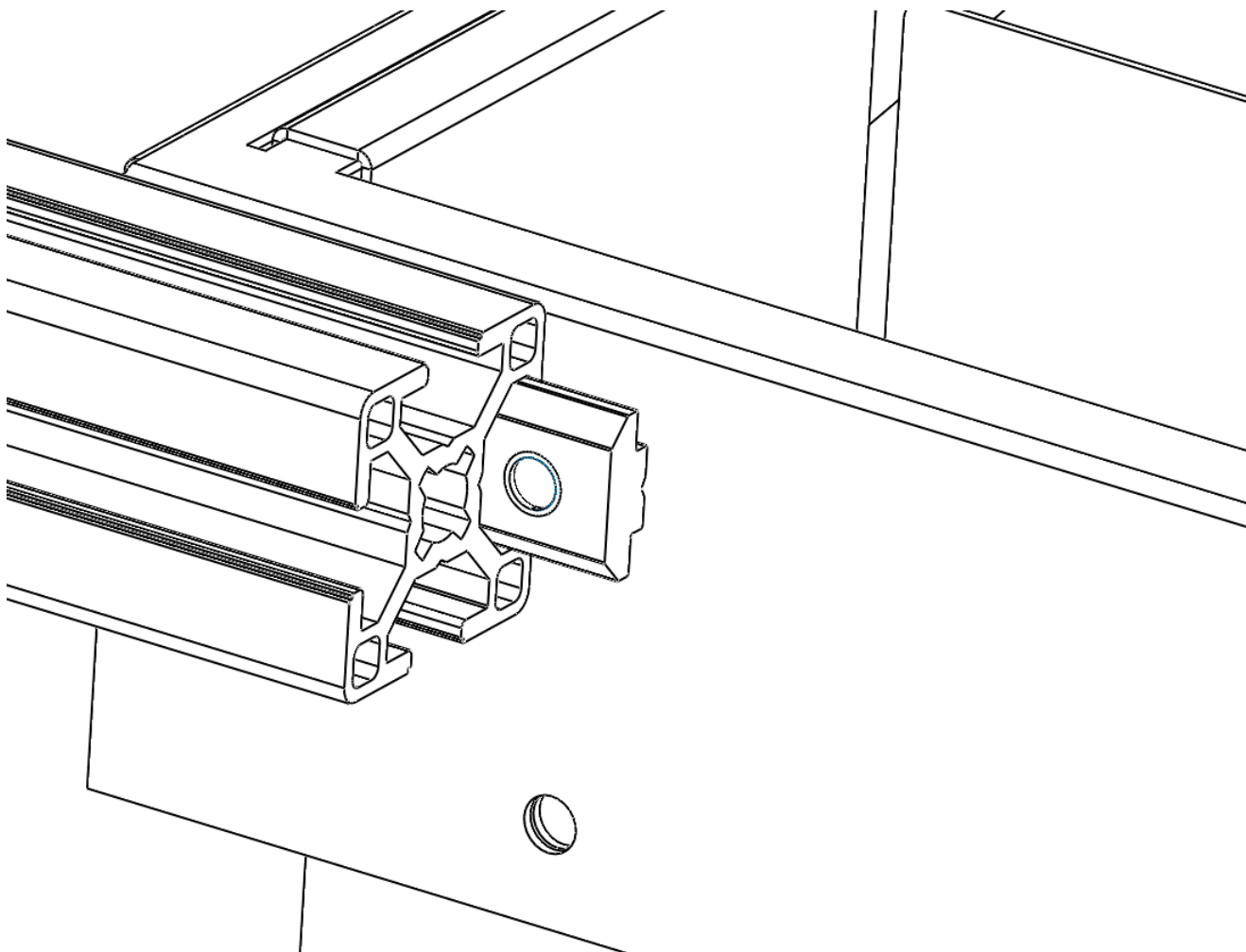
Figur 8: Monteringsdetalj för verktygsbricka
