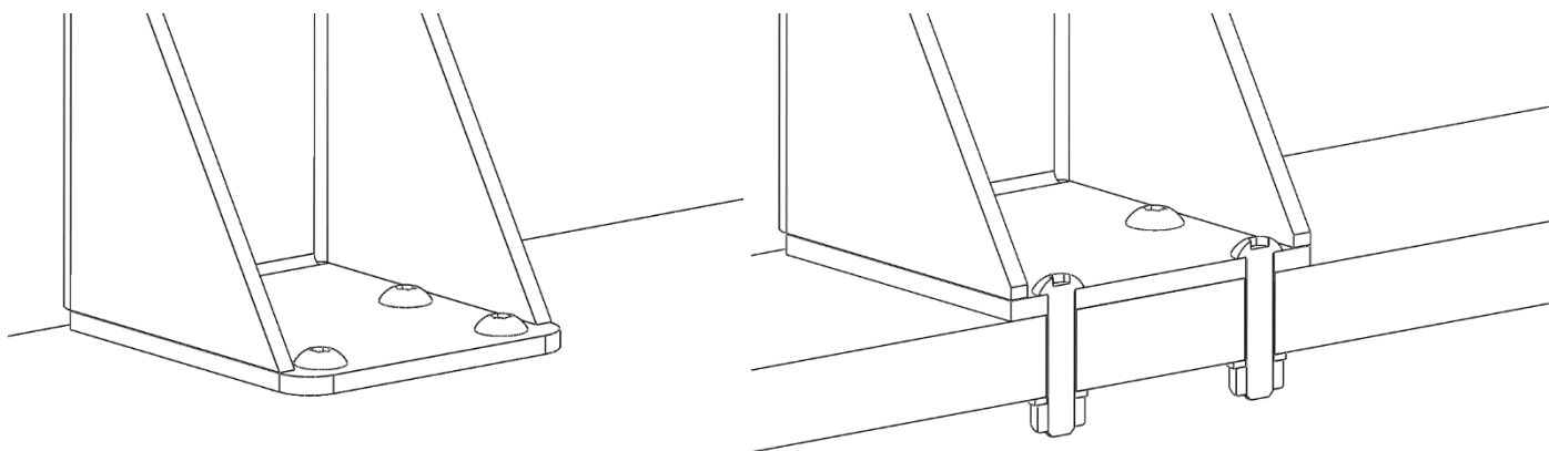
Montering med gängade skruvar / sektionsvy
