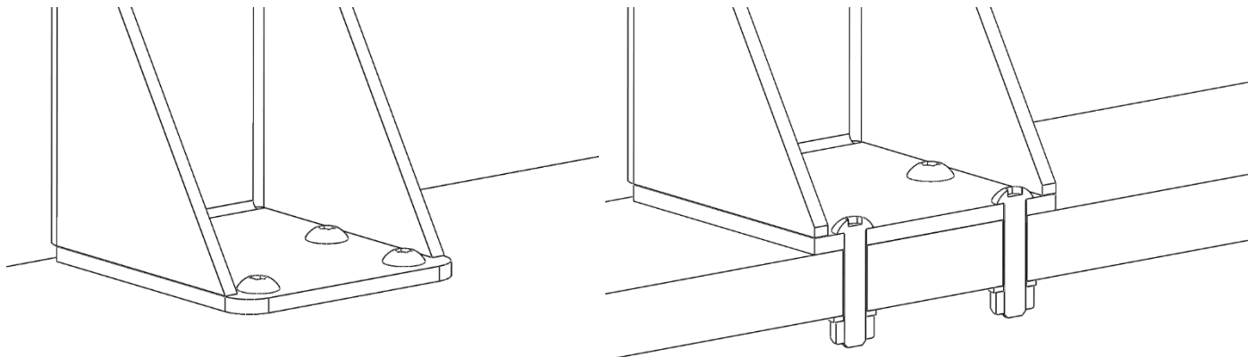
Montáž závitovými šrouby / pohled na průřez
