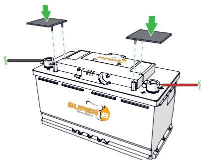
Figure 12. Positionnez les capuchons accessoires sur les terminaux de la batterie.
