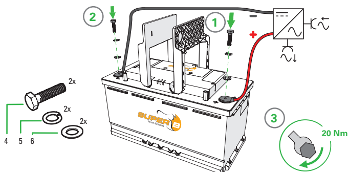
Figure 7. Connexion du raccord réducteur des câbles d'alimentation
