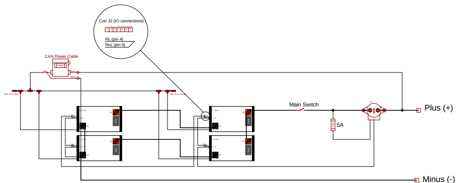
Figure 15. Vier Li-Ionen-Batterien in Serie - Parallelschaltung mit externer Abschaltvorrichtung und ohne externe Stromversorgung
