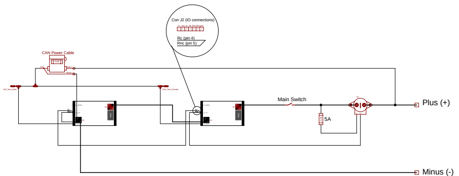
Figure 17. Verwendung des CAN-Stromkabels zur Stromversorgung des CAN-Busses
