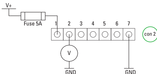
Figure 18. Bestimmung der Batterien SoC
