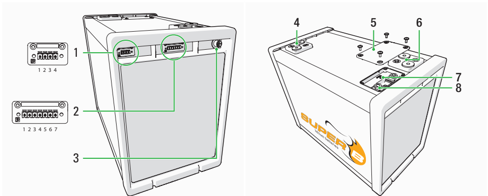
Figure 2. Anschlüsse, Anzeigen und Batteriekontrollen
