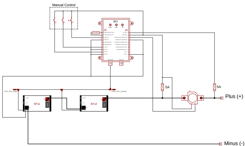
Figure 8. Anschluss einer Li-Ionen-Batterie an die SB BCI-C1
