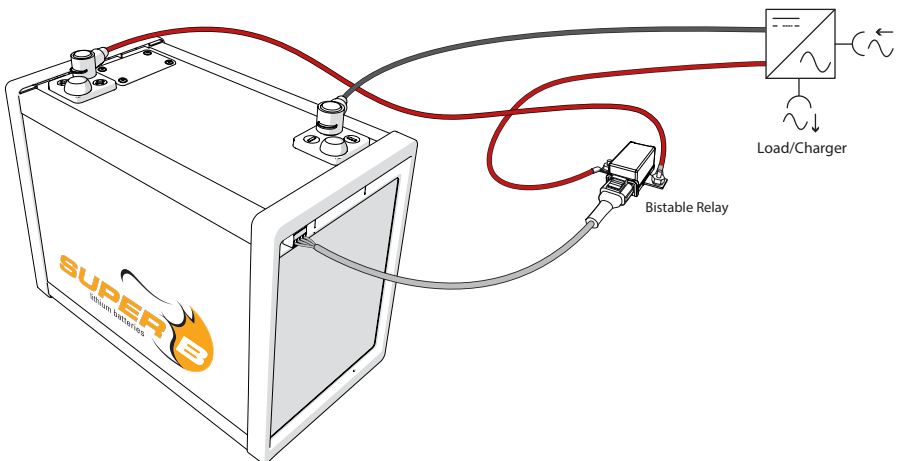
Figure 9. Abbildung 11. Anschluss der Batterie an die Last
