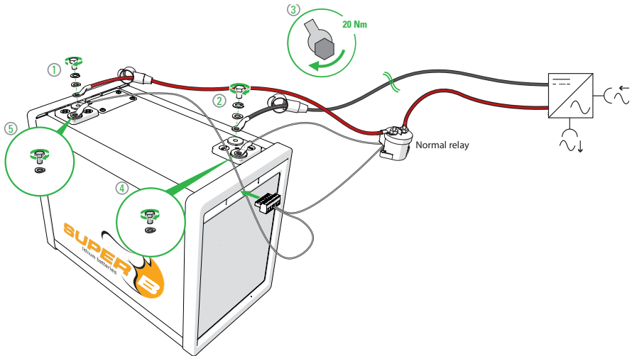
Figure 11. Anschluss der Batterie an die Last.
