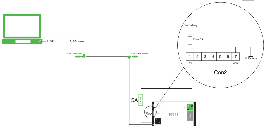
Figure 16. Verwenden Sie Con2, um den CAN-Bus mit Strom zu versorgen
