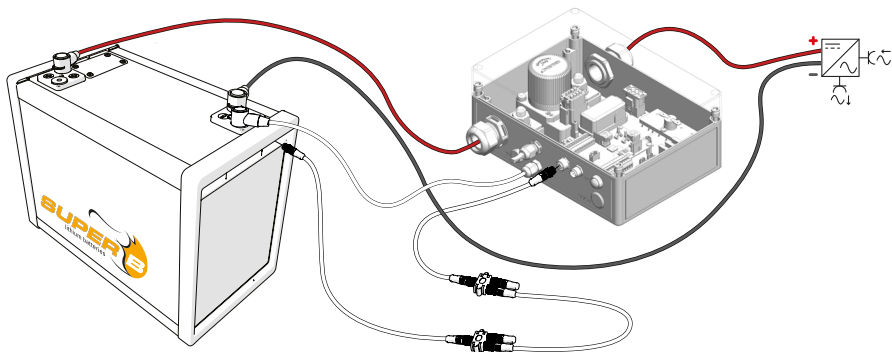
Figure 7. Anschluss einer Li-Ionen-Batterie an die SB BIB
