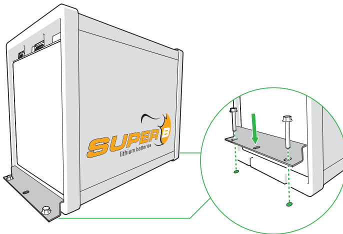
Figure 3. Abbildung 3. Installieren der Li-Ionen-Batterie mit Hilfe der Super-B-Montagehalterung
