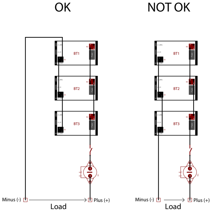
Figure 14. Drei Li-Ionen-Batterien parallel zur externen Abschaltvorrichtung
