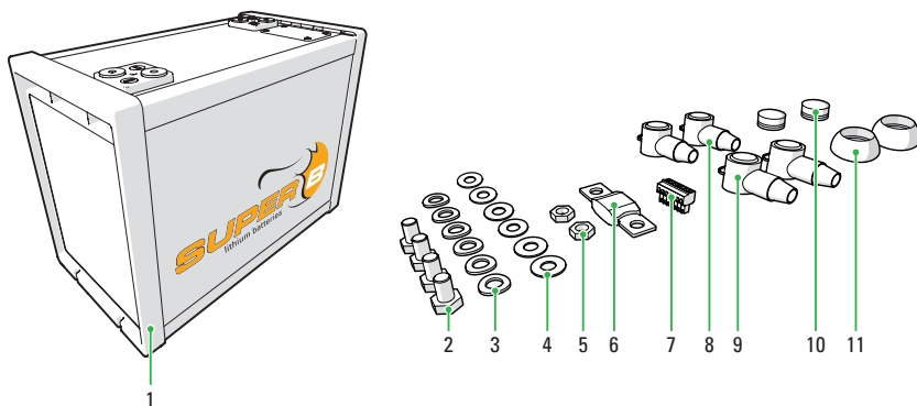
Figuur 1. Onderdelen.
