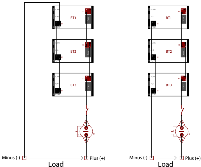
Figuur 14. Drie Li-ion accu's parallel met stroomonderbreker
