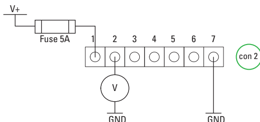
Figure 18. Détermination des SoC des batteries
