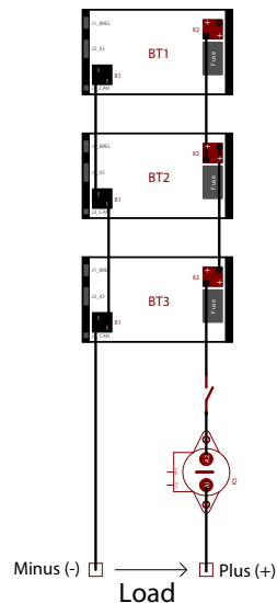
Figure 14. Drei Li-Ionen-Batterien parallel zur externen Abschaltvorrichtung
