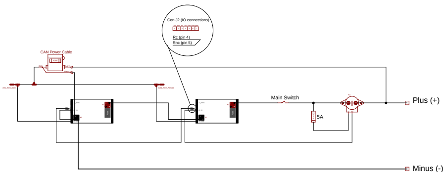
Figure 13. In Reihe geschaltete Batterien mit CAN-Netzkabel und externer Abschaltvorrichtung.
