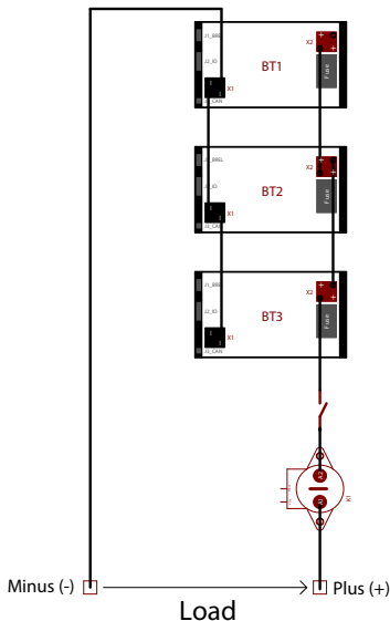
Figure 14. Drei Li-Ionen-Batterien parallel zur externen Abschaltvorrichtung
