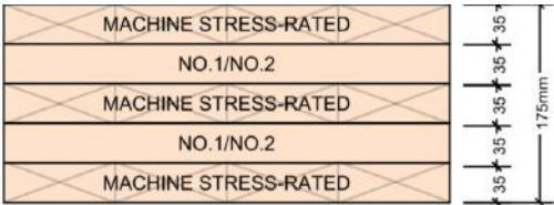
5 PLY CLT
