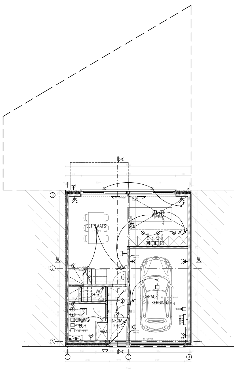
Woning 2 PLAN GELIJKVLOERS ontwerp 1/100
