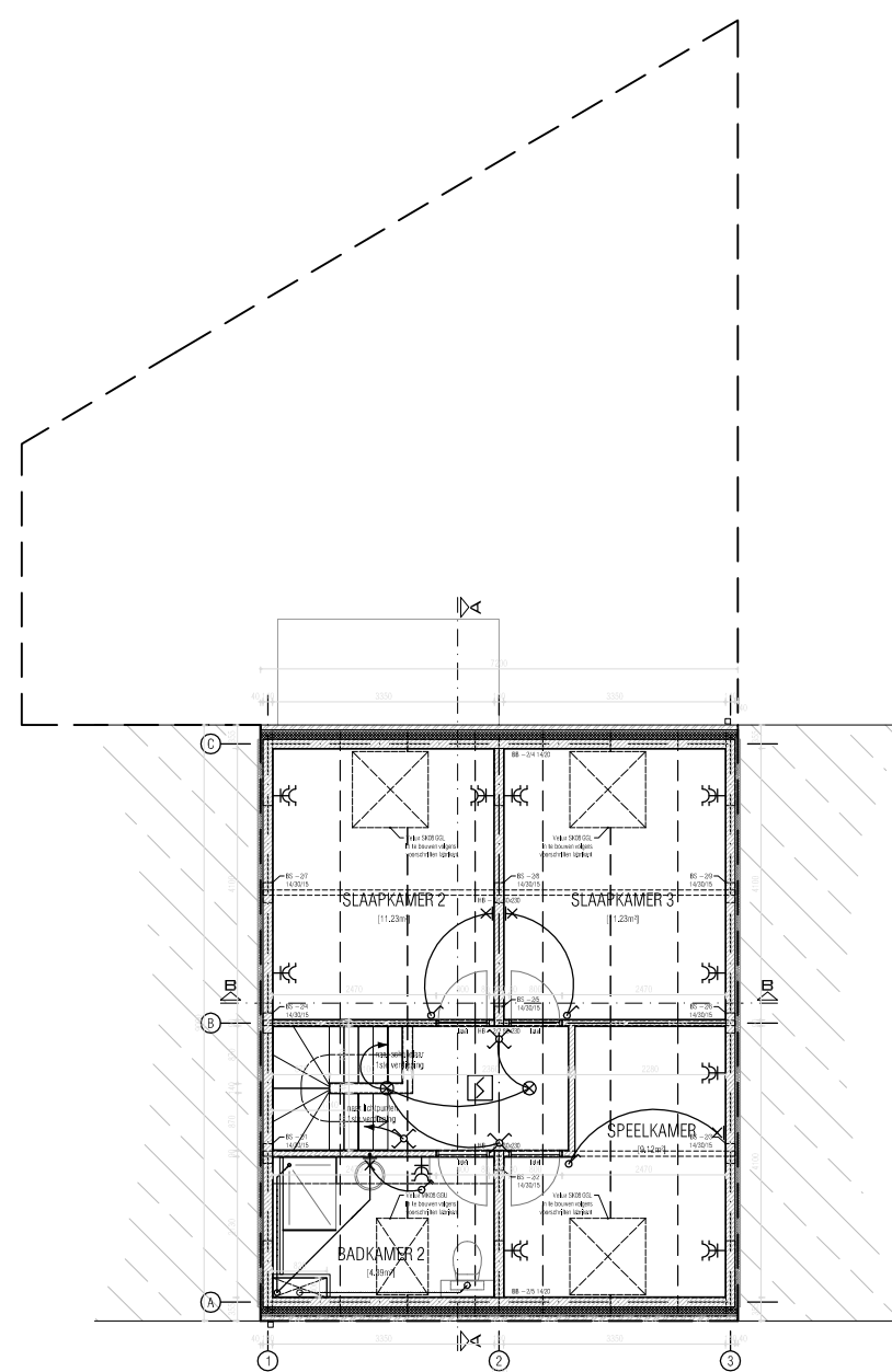
Woning 2 PLAN 2de VERDIEPING ontwerp 1/100
