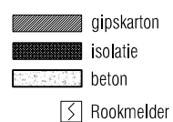
Woning 2 PLAN GELIJKVLOERS ontwerp 1/100
