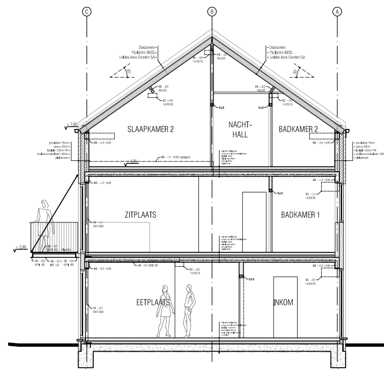
Woning 2 SNEDE A-A ontwerp 1/100
