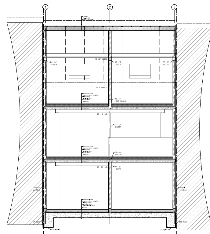
Woning 2 SNEDE B-B ontwerp 1/100
