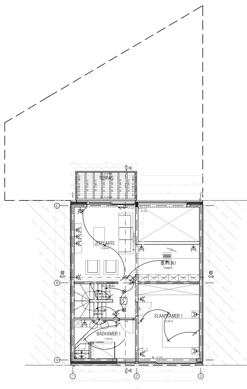
Woning 2 PLAN 1ste VERDIEPING ontwerp 1/100
