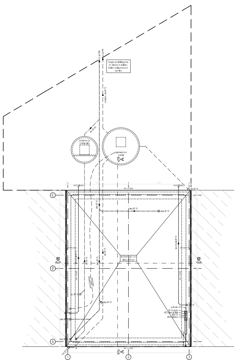
Woning 2 PLAN FUNDERING en RIOLERING ontwerp 1/100
