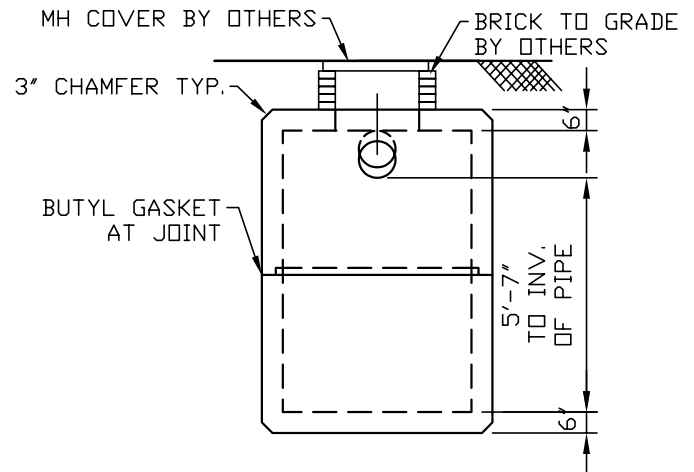
ELEVATION A-A
