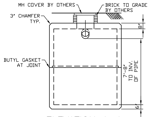
ELEVATION A-A
