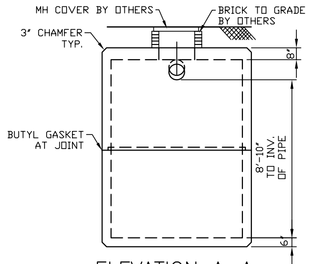
ELEVATION A-A
