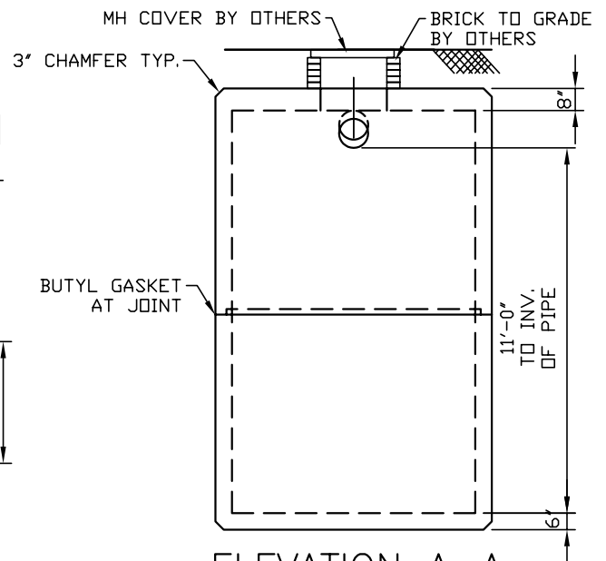
ELEVATION A-A
