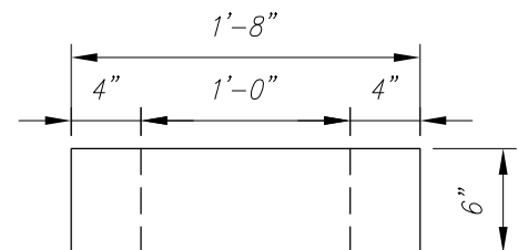
ELEVATION B-B
