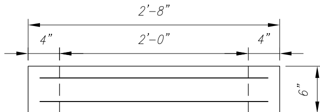
ELEVATION A-A
