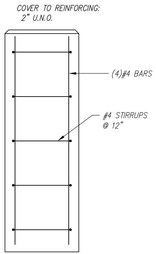
REINFORCING SECTION SCALE: N.T.S.
