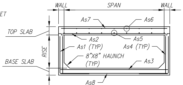
REINFORCING SECTION Scale: N.T.S.
