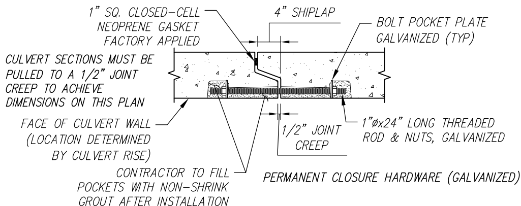
CONNECTION HARDWARE DETAIL Scale: N.T.S.
