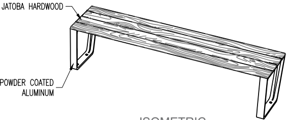
ISOMETRIC N.T.S.
