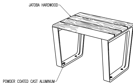
ISOMETRIC N.T.S
