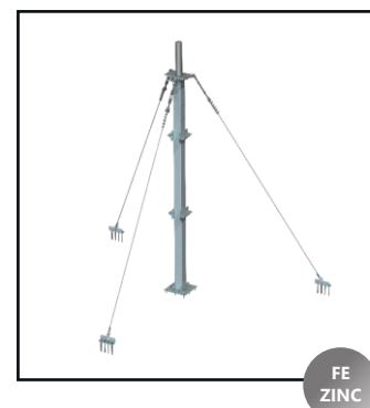
Prodotto Kit per pali da sottotetto tirantati
