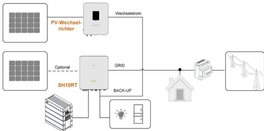
Abbildung 2-7 Backup-Anschluss zur Nachrüstung der bestehenden PV-Anlage
