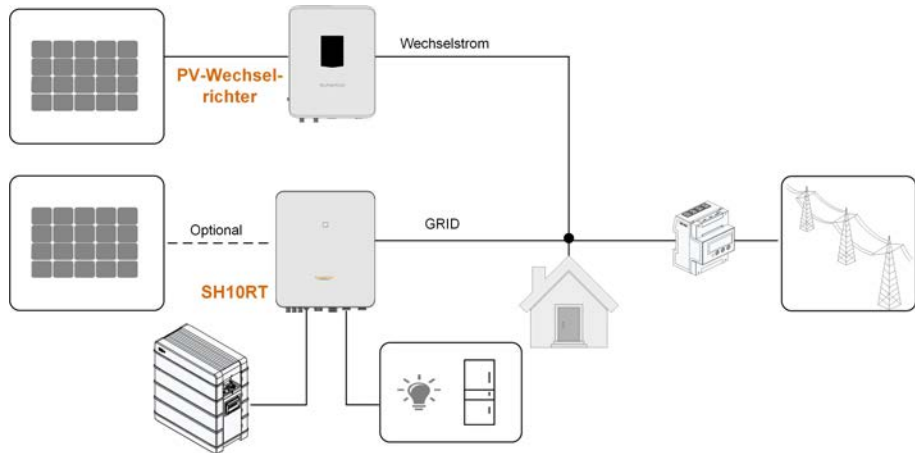
Abbildung 2-6 Netzgekoppelter Anschluss zur Nachrüstung der bestehenden PV-Anlage
