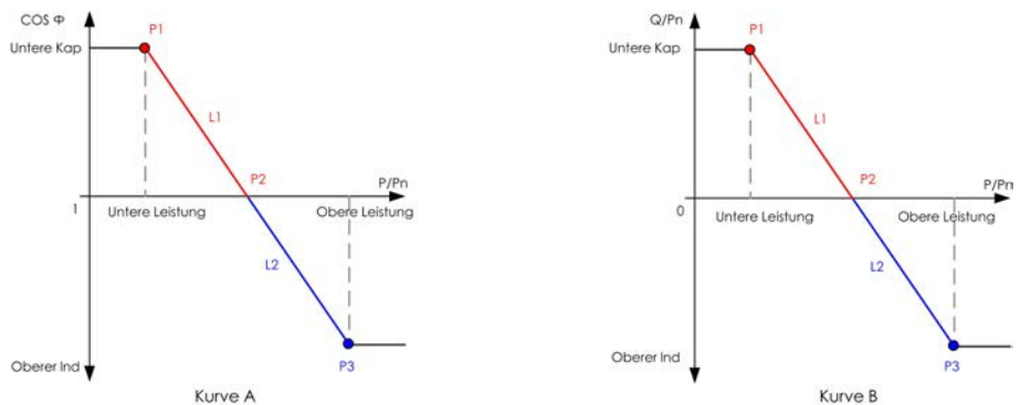
Abbildung 8-3 Q(P)-Kurve
