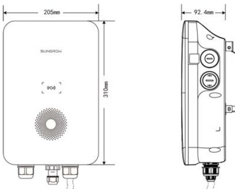
Abbildung 1-2 Abmessungen (in mm)
