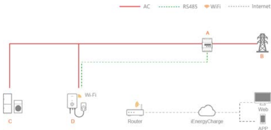
Abbildung 1-5 Systemtopologiediagramm Lastausgleich
