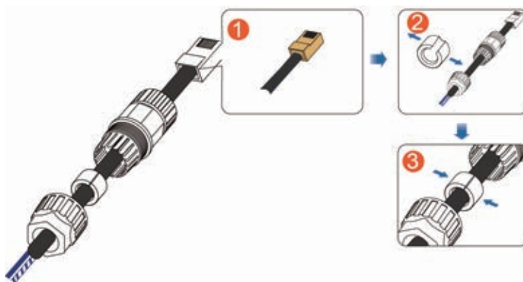
Abbildung 2-3 RJ45-Schraubanschluss (B)
