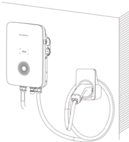
Abbildung 2-6 An der Wand montierte Ladestation
