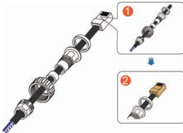
Abbildung 2-2 RJ45-Schraubanschluss (A)
