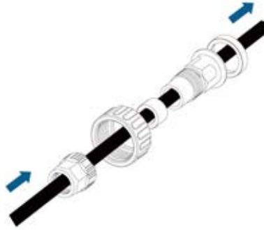
Abbildung 2-2 RJ45-Komponenten
