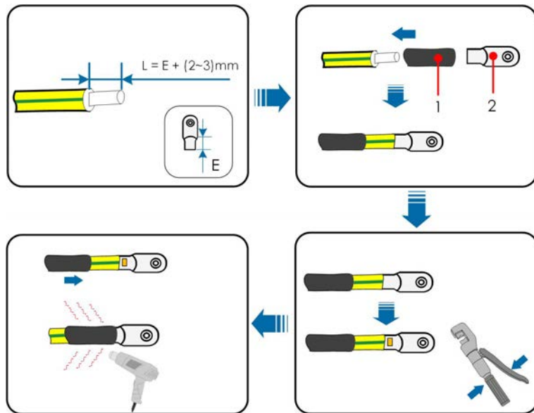
(1) Schrumpfschlauch
