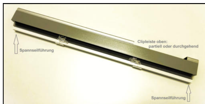
(2) Interial® I-06 Modell 1S mit Clipleiste und Seilführung
