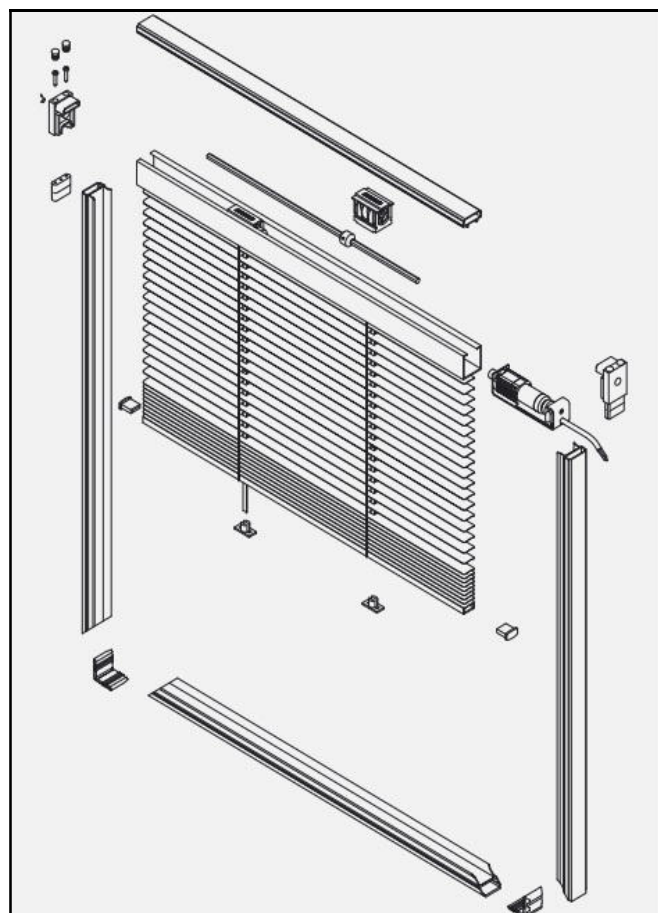
Interial® Modell 1 Vollfunktion mit Motorantrieb im Rahmen
