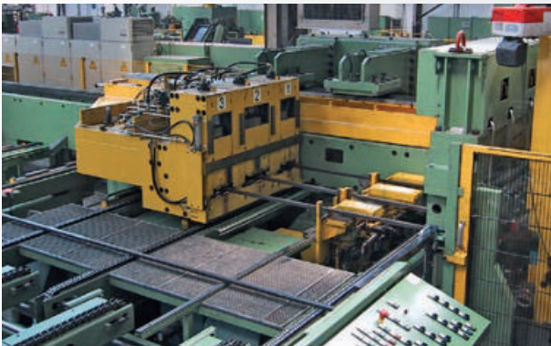
3-fach-Stangenziehanlage für Stahlstangen mit Einschubvorrichtung Triple drawing line for steel bars with push-in device
