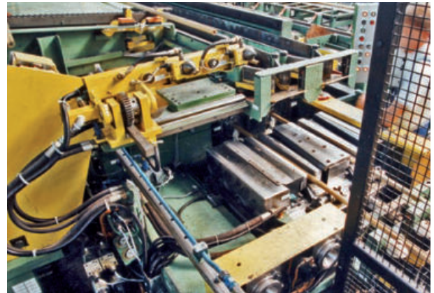
2-fach-Einschubvorrichtung in einer 2-fach-Stangen- und Profildrehmaschine für Messingstangen Double push-in device within a double drawing machine for brass bars and profiles
