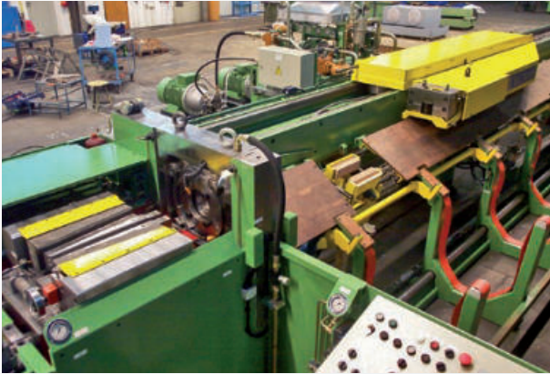
1-fach-Stangenziehanlage für Messingstangen mit Einschubvorrichtung Single drawing line for brass bars with push-in device
