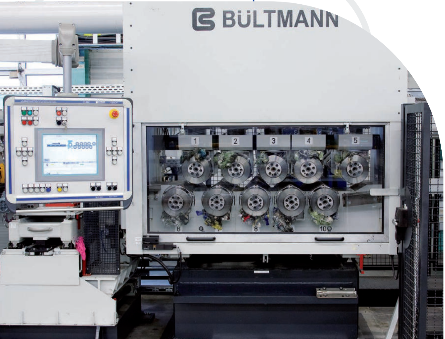
2 x 10-Rollen-Richtmaschine für Messingstangen, mit lagerichtiger Zufuhr der zu richtenden Stangen 2 x 10-roll straightening machine for brass bars, with feeding of bars in correct position
