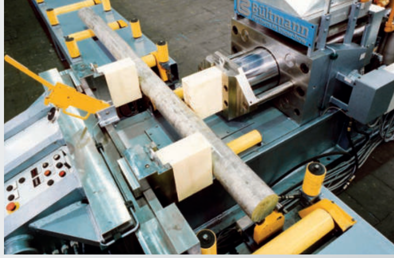
3000 kN Richtpresse für Aluminiumstangen und -profile 3000 kN straightening press for aluminium bars and profiles
