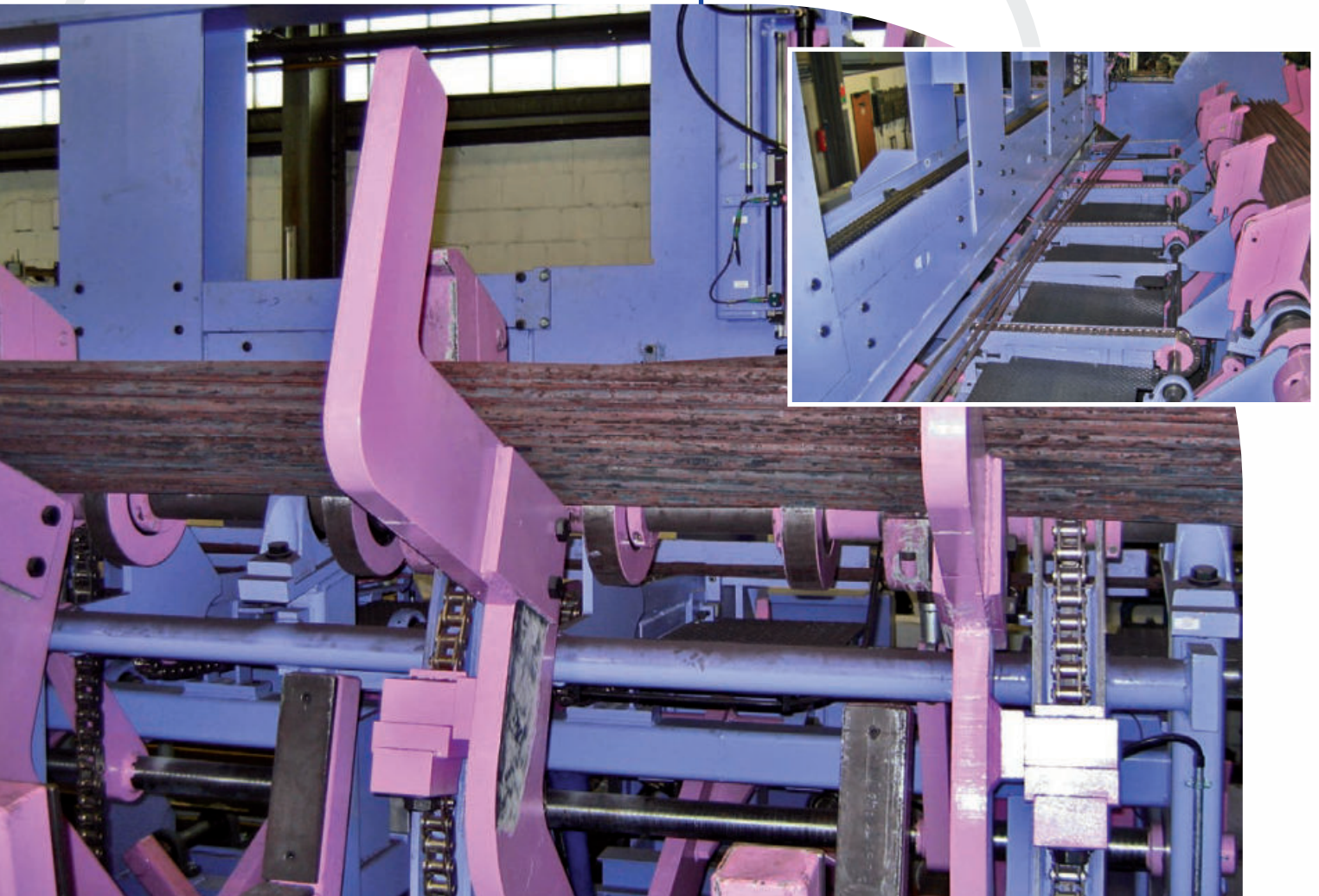
Stangenvereinzlung vor einer Richtmaschine für schwarze Rundstangen Separation system in front of a straightening machine for round black bars
