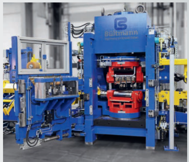
2-Walzen-Richt- und Poliermaschine für geschälte Stangen 2-roll straightening/polishing machine for peeled bars
