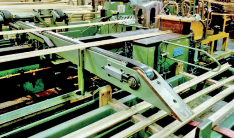
Reckanlage mit Entdrallkopf für Messingstangen und -profile Stretching line with detwisting device for brass bars and profiles
