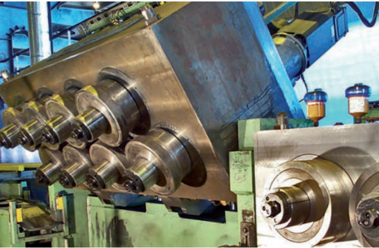
2 x 8-Rollen-Richtmaschine für Stahlstangen und Flachmaterial 2 x 8-roll straightening machine for steel bars and flats
