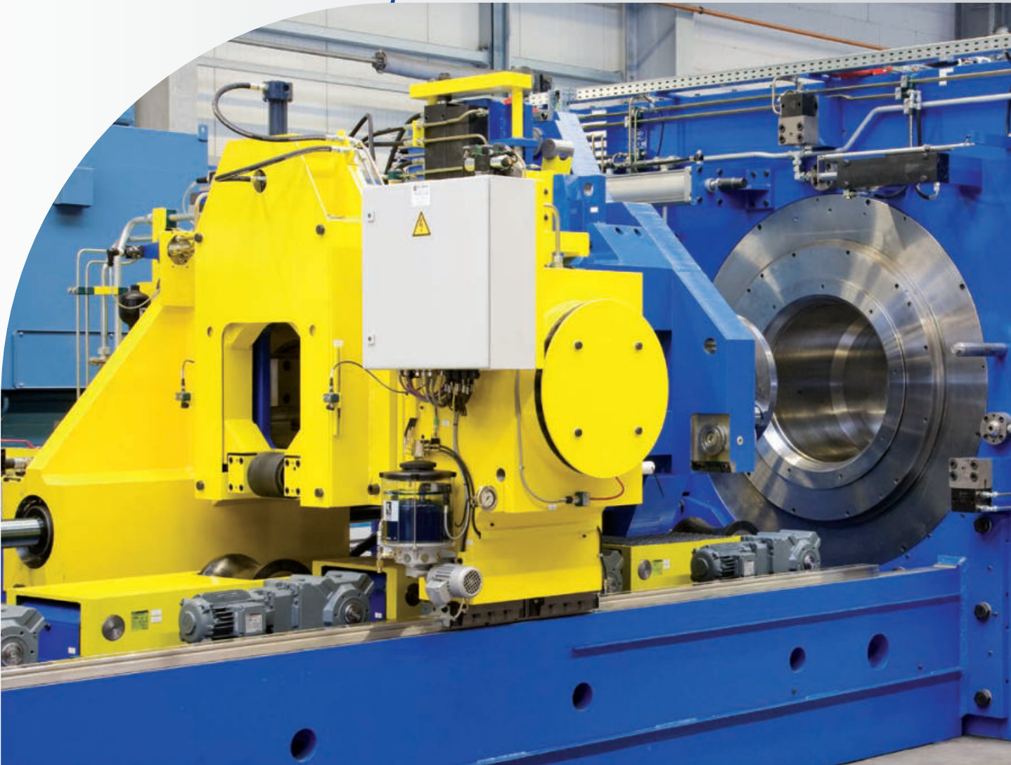
Auszugswagen einer Schälmaschine für Edelstahlstangen Extraction carriage of a peeling machine for special steel bars
