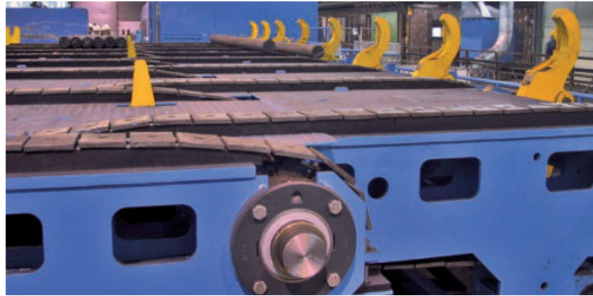
Stangenvereinzlung vor einer Schälmaschine bis Stangendurchmesser 320 mm Bar separation system in front of a peeling machine up to a bar diameter of 320 mm
