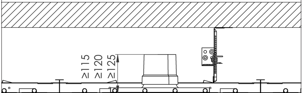
Lüftungshaube Breeze mit Anschlussstutzen / Diffuser Breeze with connection piece/ Diffuseur Breeze avec raccordement droit
