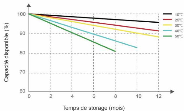
Courbe d'autodécharge selon différentes températures
