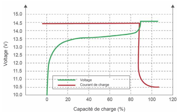
Caractéristiques de charge (0.5°C, 25°C)
