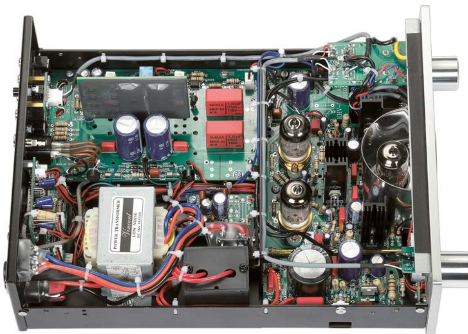
Trotz hoher Bauteilverdichtung gibt es keine Thermik-Probleme der Röhren.
