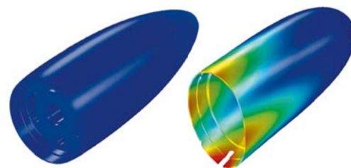
Das aus der 800er-Baureihe abgeleitete Aluminiumgehäuse des Hochtöners (links im Bild) ist viel stabiler als der Vorgänger. Resonanzen, wie das Wärmebild zeigt, werden erheblich besser bedämpft.
