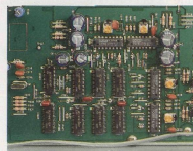
harman/kardons „Real-Time Linear Smoothing“ funktioniert über eine Kette von Speicherchips mit herkömmlicher Wandlertechnologie.
