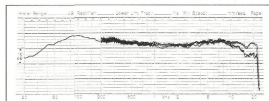
Frequenzgang der linken und rechten Box auf Achse und jeweils 40 Grad nach außen gedreht. Unter 200 Hz Nahfeld
