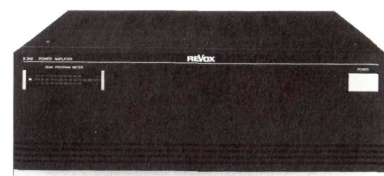
Energiestation: Die neue Endstufe B 242 liefert zwei mal 200 Watt an vier Ohm
