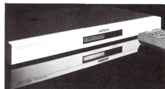
Eine Menge Komfort-Zuwachs bringt der Timer-Controller B 203 für denjenigen, dessen HiFi-Anlage aus Revox-Komponenten besteht. Bis zu acht Bausteine lassen sich anschließen
