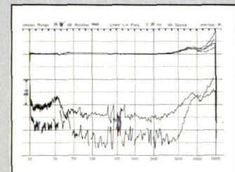
Sony XL-MC 3: Frequenzgang und Übersprechen
