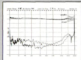
Braun MC-2 E: Frequenzgang und Übersprechen
