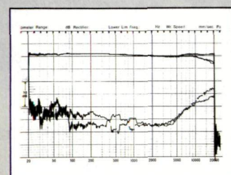
Denon DL-110: Frequenzgang und Übersprechen
