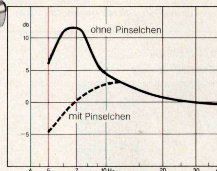
3. Dämpfende Wirkung des Dustomatic-Pinzelchens auf die Tonarmresonanz.
