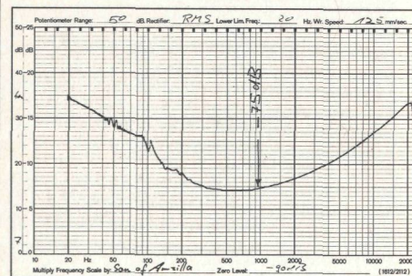
Die Übersprechdämpfung zwischen den Stereokanälen beim Son of Ampzilla
