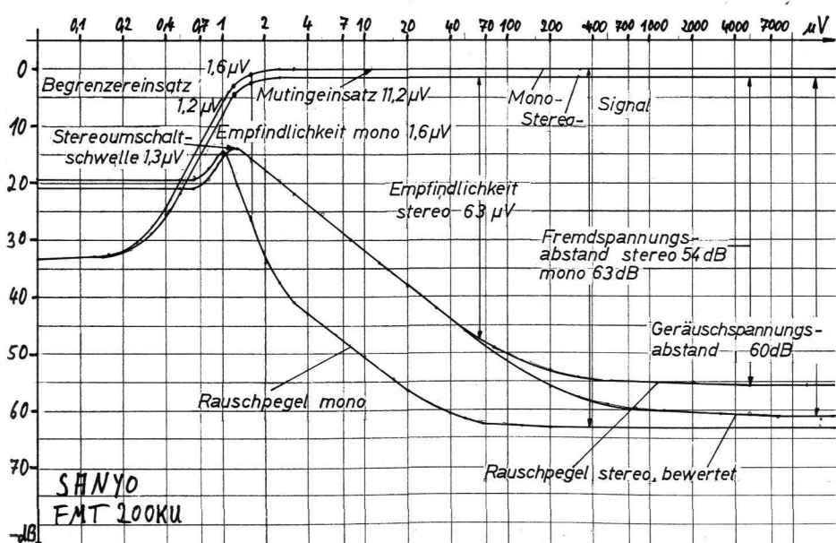
Tunerteil vom 300-Ohm-Antenneneingang bis zum Tonbandausgang gemessen mit 40 kHz Hub.
