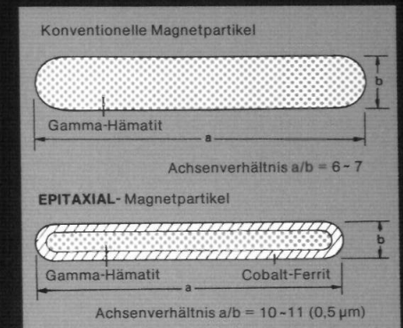
Struktur des Magnetmaterials
