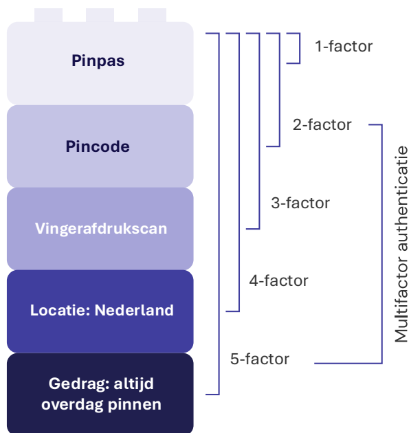
Afb. 1: Multifactor authenticatie.
