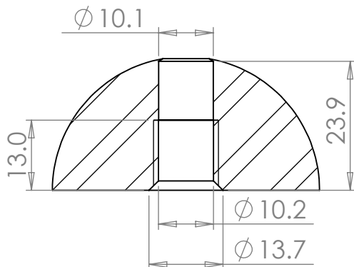
SECTION D-D
